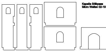
Wandteile/wall parts
